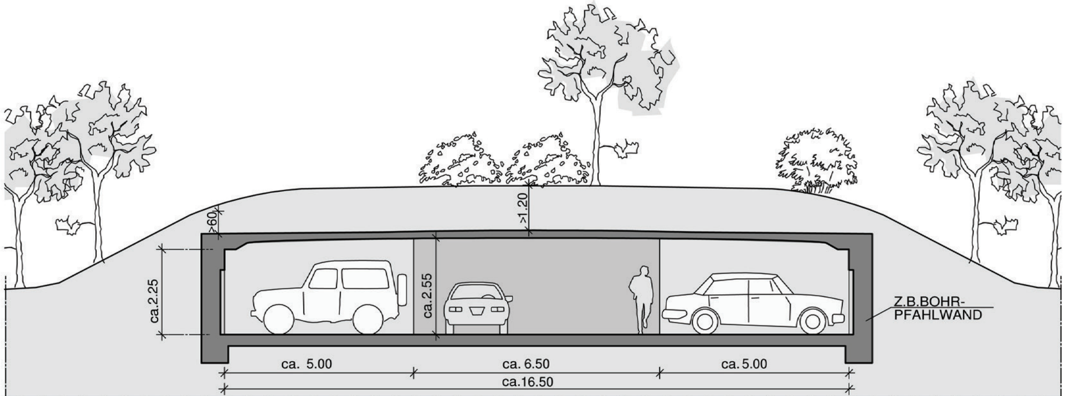
Skizze Querschnitt Vorschlag Variante 1, M.1:100
